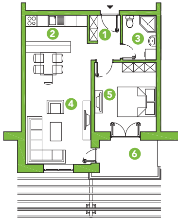
Apartman 4
