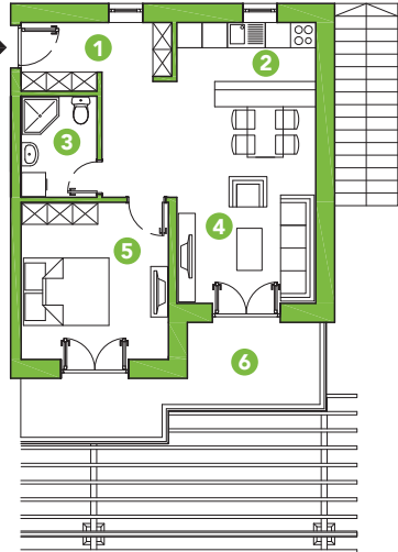
Apartman 5
